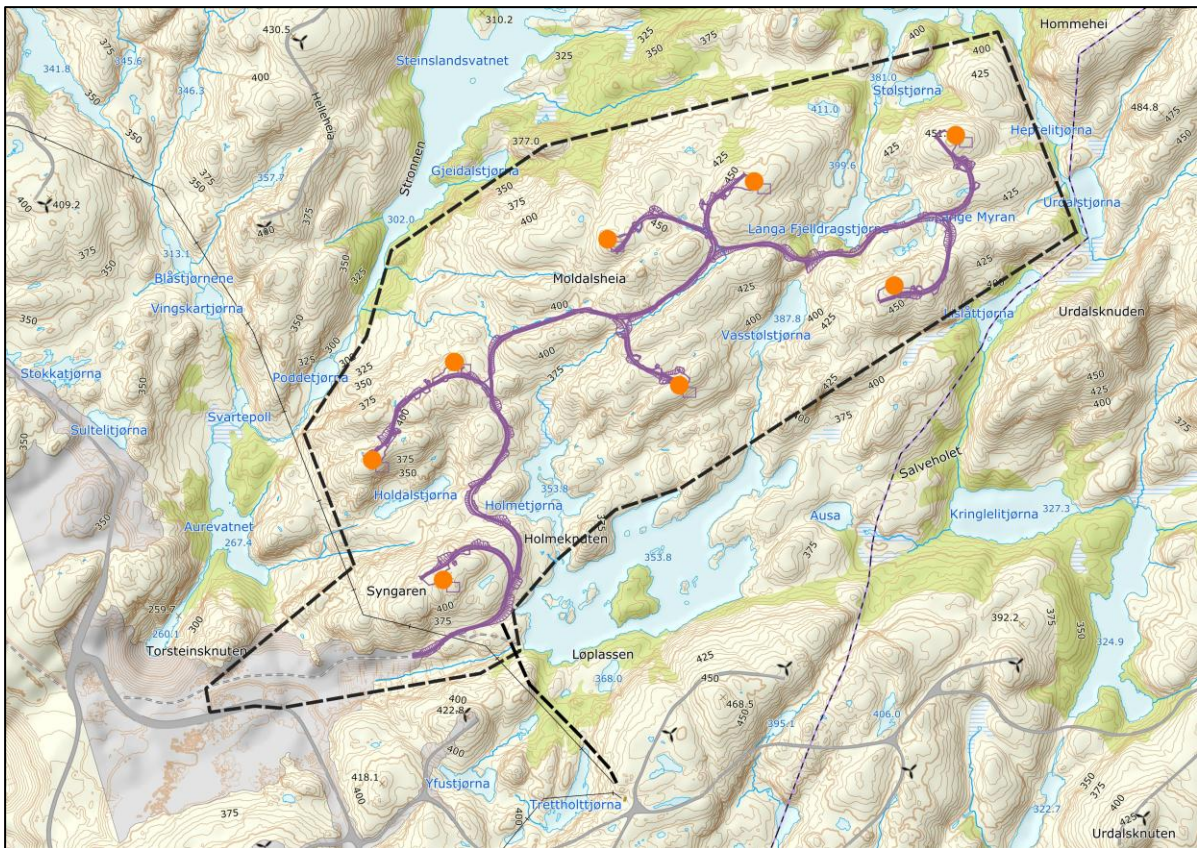
Figur 2.5. Layout A – 8 turbinposisjoner
