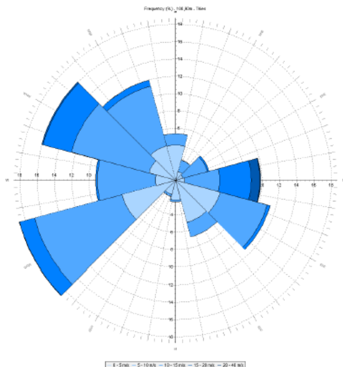
Figur 6.1. Vindrose for telledagene, basert på data fra målemasta (fra Meventus). Lengden på kjeglene står for frekvens. De lyseste blåfargene viser de roligste vindforholdene.
