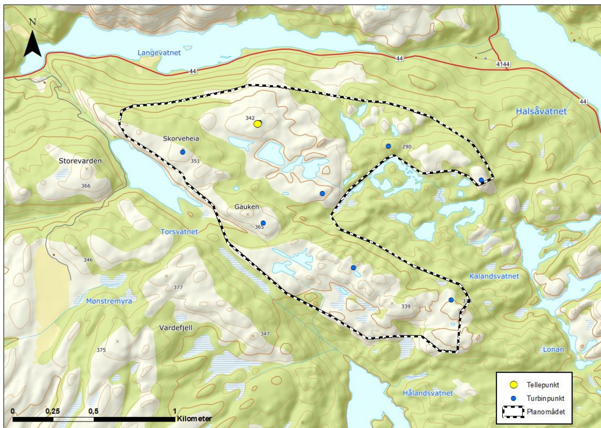
Figur 5.1. Beliggenhet av tellepunktet for rovfugltellingene høsten 2019.
