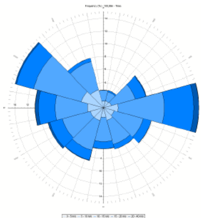
Figur 6.3. Vindrose basert langtidskorrigererte data for perioden 10.8-10.11 1999 – 2019 (fra Meventus). Lengden på kjeglene står for frekvens. De lyseste blåfargene viser de roligste vindforholdene.
